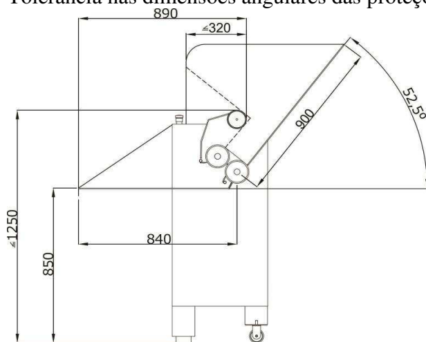
Legenda - dimensões em milímetros com tolerância de 25,00 mm (vinte e cinco milímetros) Figura 2: Desenho Esquemático com as distâncias de segurança do cilindro soador.
