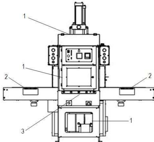
Figura 22: Máquina de alta frequência com corte hidropneumática/hidráulica com deslocamento automático da mesa - Vista frontal
